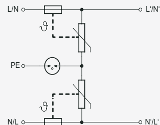
Схема принципова
